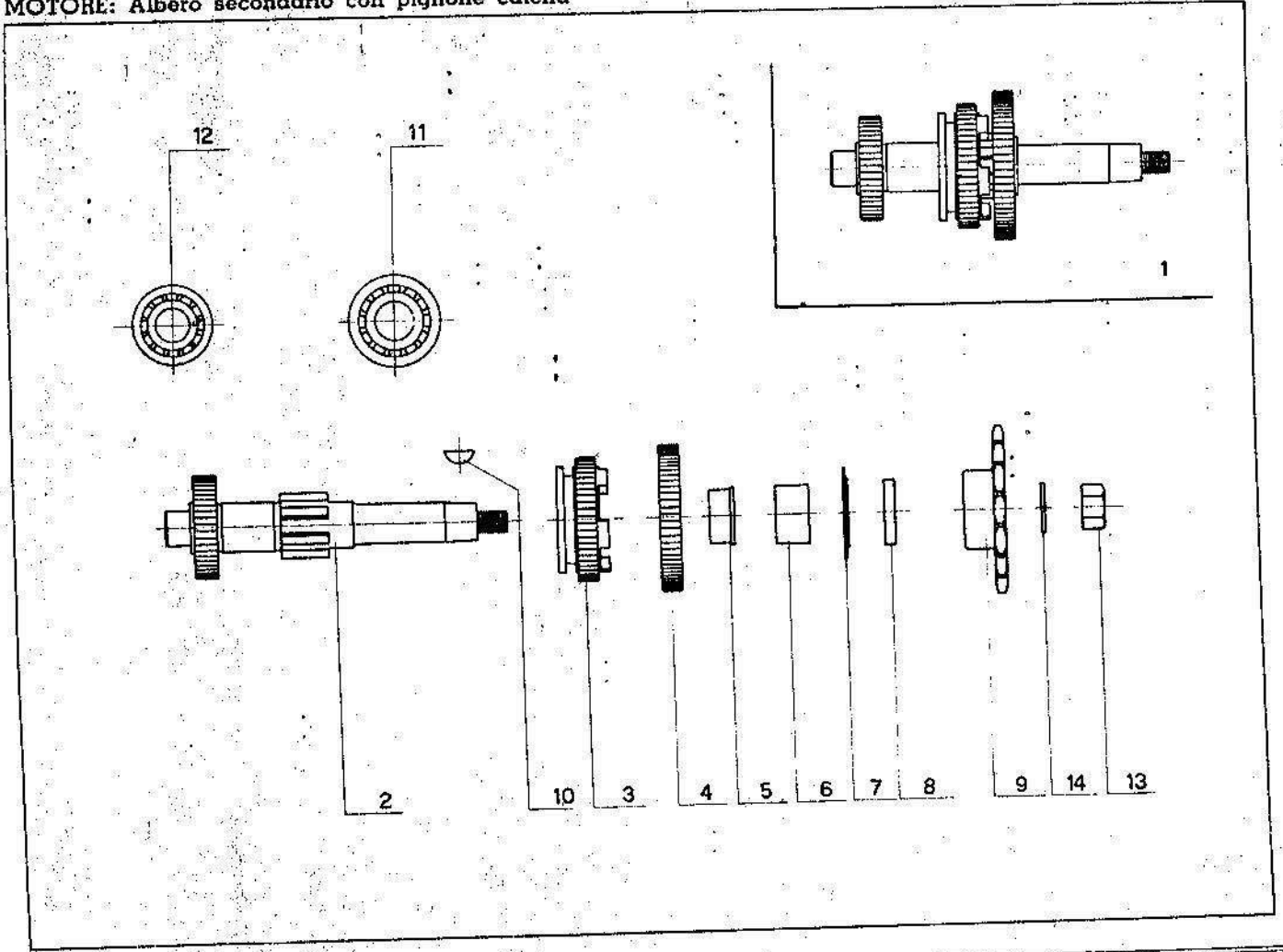
MOTORE: Albero secondario con pignone catena
